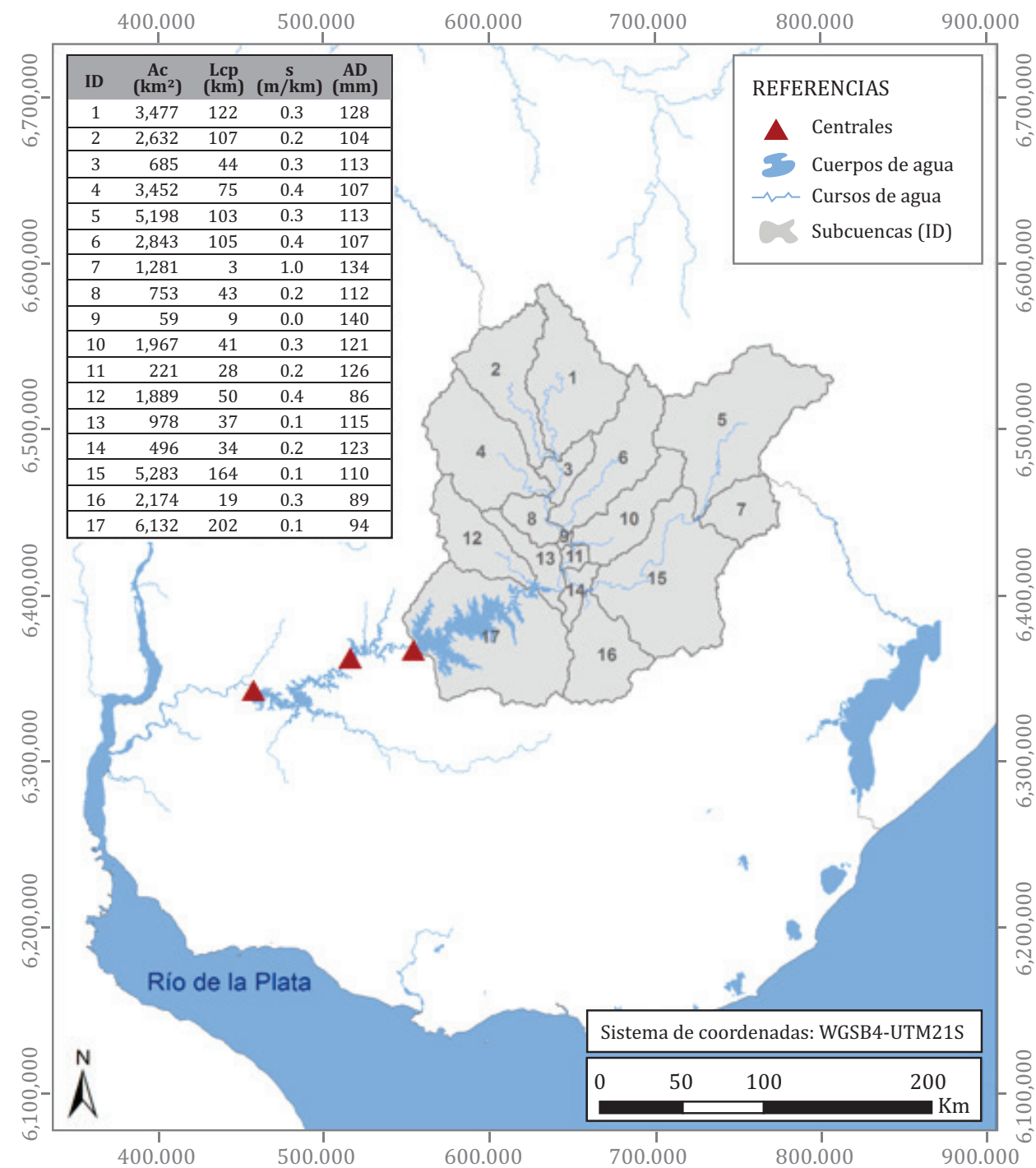
Figura 3. Discretización en subcuencas de la cuenca de aporte a Rincón del Bonete. Se incluye una tabla con el área de la cuenca de aporte (km 2 ), la longitud (km) y pendiente media (m/km) del cauce principal y al agua disponible ponderada (mm) de cada subcuenca (identificada según un ID).
