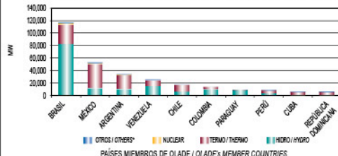
CAPACIDAD INSTALADA PARA GENERACIÓN ELÉCTRICA POR TIPO DE PLANTA INSTALLED CAPACITY FOR ELECTRICITY GENERATION BY TYPE OF PLANT
