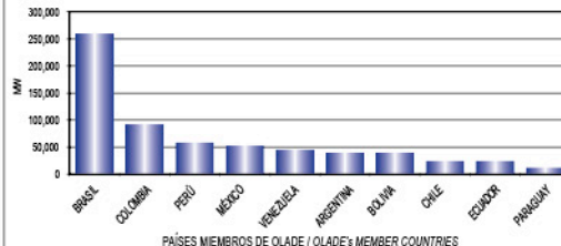
POTENCIAL HIDROELÉCTRICO AL&C HYDROPOWER POTENTIAL LA&C
