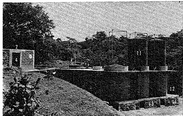
Fig. 17. Entre la batería de silos (9) y las pilas de los gasómetros (11), se encuentra la sala de administración (10), en la que funciona un generador de 1 Kwh, accionado por biogas, para la iluminación de toda la planta y casa del administrador; un poste de compresión, un filtro para el gas y control general de la línea de gas.
