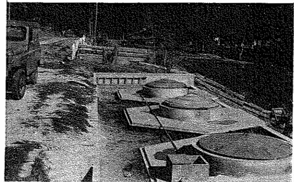
Fig. 7. La misma planta "La Sierra" vista por arriba, mostrando su estructura y diseño. Izq. camino de acceso para carga y descarga; Cen. las cámaras y sus cubiertas, dos son fibra de vidrio; Der. frente, patio de descarga y decantación; Der. fondo, un alfalfar creceolozano con bioabono.
