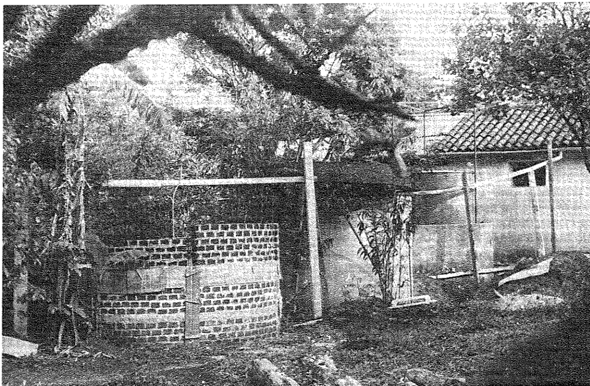
Fig. 2 Primera Planta Piloto de Biogas, construída en la ciudad de Guatemala, 1953. Capacidad de cada cámara 10 Tons. Gasómetro metálico calculado 10 grs/cm 2 . Izq. cámara en construcción; cent. cámara en funcionamiento; der. gasómetro. Datos en Cuadro No. 1
