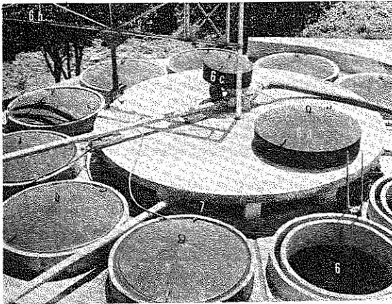
Fig. 14. Batería de diez tanques de fermentación, en cuyo centro se encuentra el cuarto de bombeo y trasiego (7). La cámara (6) se está descargando, luego de quitar su tapadera (6a), por medio del puente giratorio (6b).
