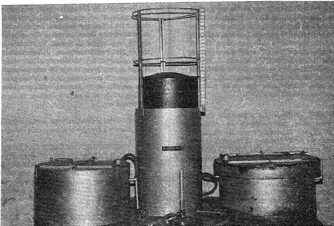
Fig. 1. Primera Planta de Biogas, construída en Guatemala en el año de 1952. Capacidad de cada fermentador 4-litros Gasómetro metálico calculado 5 gr/cm 2 .
