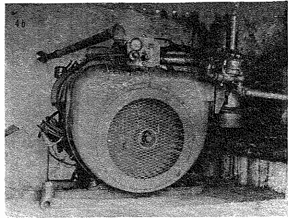
Fig. 13. Este motor situado en (4b), es marca "Wisconsin", con 35 H.P. de potencia y es el que por más de 15 años ha accionado el Molino de la Planta, consumiendo parte del gas biológico producido.
