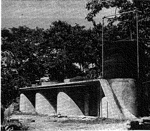
Fig. 3. Planta San Alberto, primera Planta fija montada en una finca para el aprovechamiento del estiércol de 12 vacas estabuladas y la pulpa de café del beneficio húmedo. Ver Cuadro No. 1.
