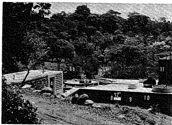
Fig. 10. Vista lateral de la planta completa.
