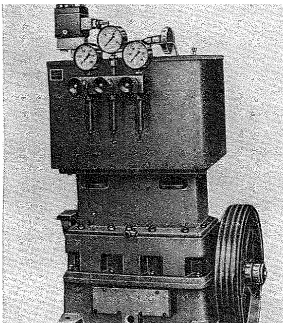
Fig. 18. Este es el compresor de alta presión, 3 etapas, modelo D 160, marca "Antillas", que comprime el biogas a 200 Kgs/cm 2 ., en cilindros de acero con capacidad para 53 litros de agua y con un contenido de 13.25 m 3 . de biogas. Es accionado por un motor de cuatro tiempos, accionado a gas, marca "ILO". Una instalación de embotellamiento para llenar seis cilindros/día.
