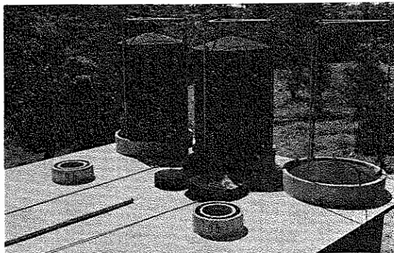
Fig. 16. Batería de gasómetros para la captación del gas y que han sido calculados para darle la presión de utilización en los diferentes motores. Compuesta de tres gasómetros, con capacidad de 15 m 3 . cada uno. Los dos de la izquierda captan el biogas de la batería (6); el de la derecha, el gas que producen los líquidos en la batería de silos (9). En (9b), pueden verse las aberturas de sello, que dan acceso a mantenimiento. Estos silos son cargados y descargados por medio de la bomba de lodos.
