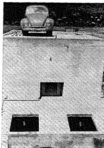
Fig. 11. Vista frontal del patio de descarga terraza superior (3) y cuarto molienda en (4), en (5) dos de los tanques prefermentadores.
