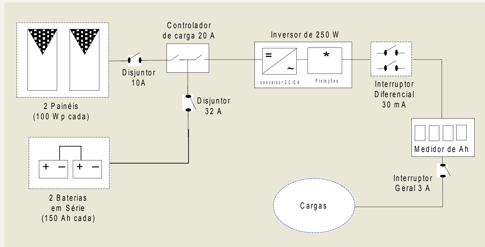
Figura 3 – Diagrama de SIGFI 13. Fonte: LSF/IEE/USP 2011
