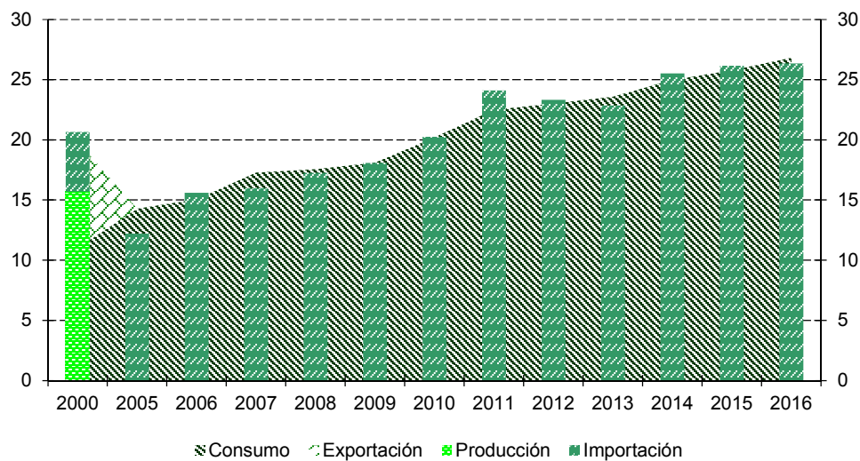
GRÁFICO 24 PANAMÁ: BALANCE DE DERIVADOS DEL PETRÓLEO, 2000, 2005-2016 (En millones de barriles)
