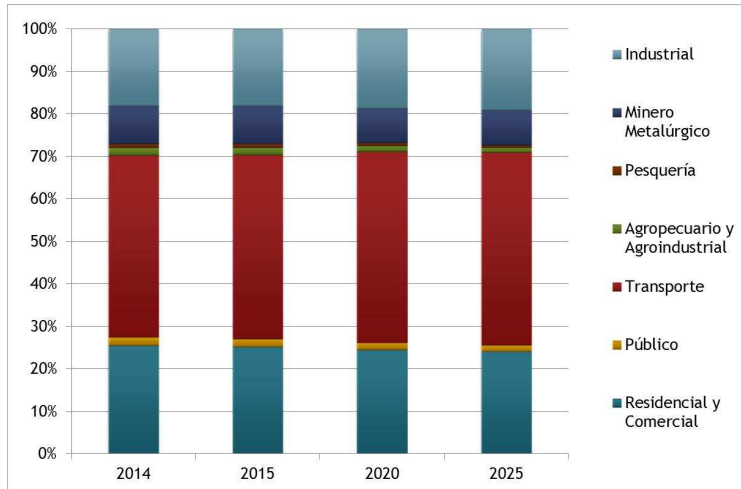
Gráfico 46 Estructura de la participación del Consumo Final de Energía por sectores. Escenario: PBI 4,5%
