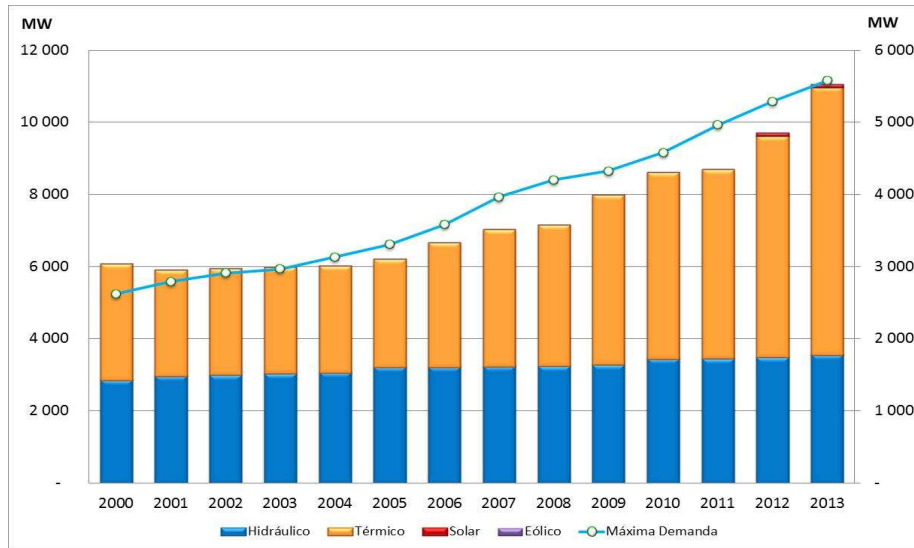
Gráfico 19 Potencia Instalada vs Demanda
