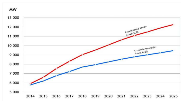
Gráfico 63 Proyección de la Máxima Demanda 2014-2025
