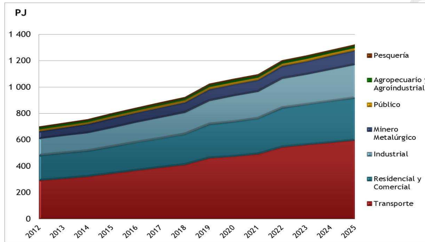
Gráfico 44 Evolución del Consumo Final de Energía por sectores 2014-2025 Escenario: PBI 4,5%
