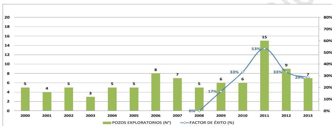
Gráfico 29 Evolución del N° de Pozos Exploratorios y Factor de Éxito
