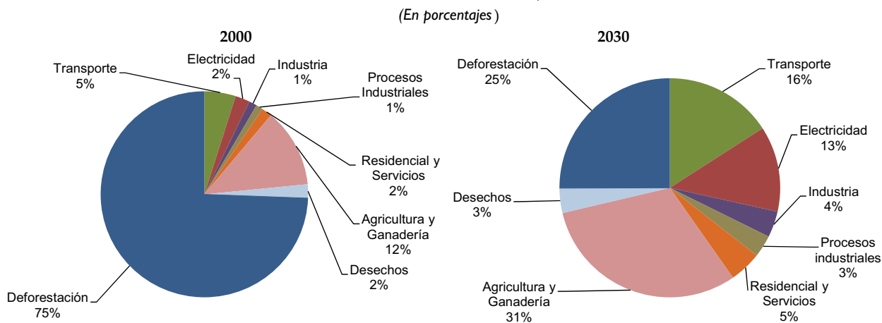
GRÁFICO 11.6 CENTROAMÉRICA: ESTRUCTURA SECTORIAL DE LAS EMISIONES DE GEI ESTIMADAS CON CAMBIO DE USO DE TIERRA, 2000 Y 2030
