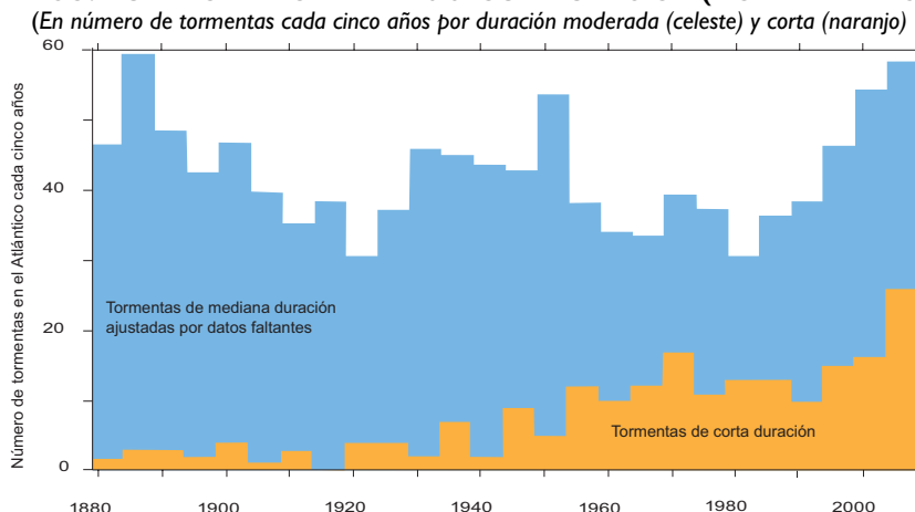
GRÁFICO 7.5 OCÉANO ATLÁNTICO: NÚMERO DE TORMENTAS SEGÚN DURACIÓN (MODERADA Y CORTA), 1878-2006
