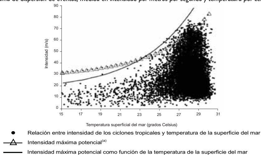
GRÁFICO 7.6 OCEANO PACÍFICO: INTENSIDAD DE CICLONES Y TEMPERATURA DE LA SUPERFICIE DEL MAR (Diagrama de dispersión de eventos, medida en intensidad por metros por segundo y temperatura por centígrados)
