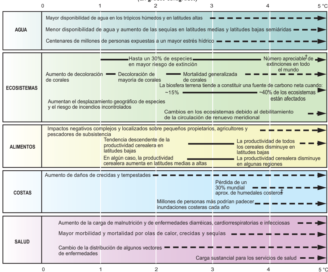
FIGURA I.1 CAMBIO ANUAL MEDIO MUNDIAL DE LA TEMPERATURA, 1980 - 1999 (En grados centígrados)
