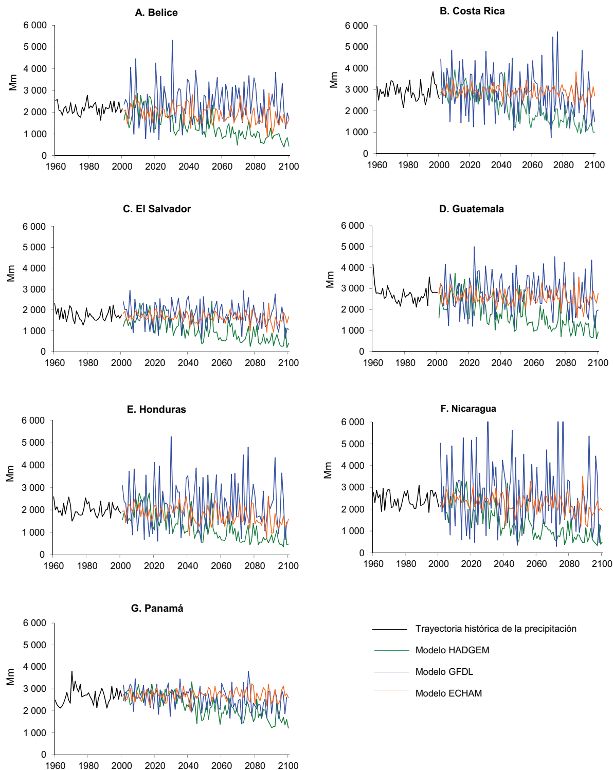
GRÁFICO 1.2 CENTROAMÉRICA: PRECIPITACIÓN ACUMULADA ANUAL, ESCENARIO A2, 1960-2100
