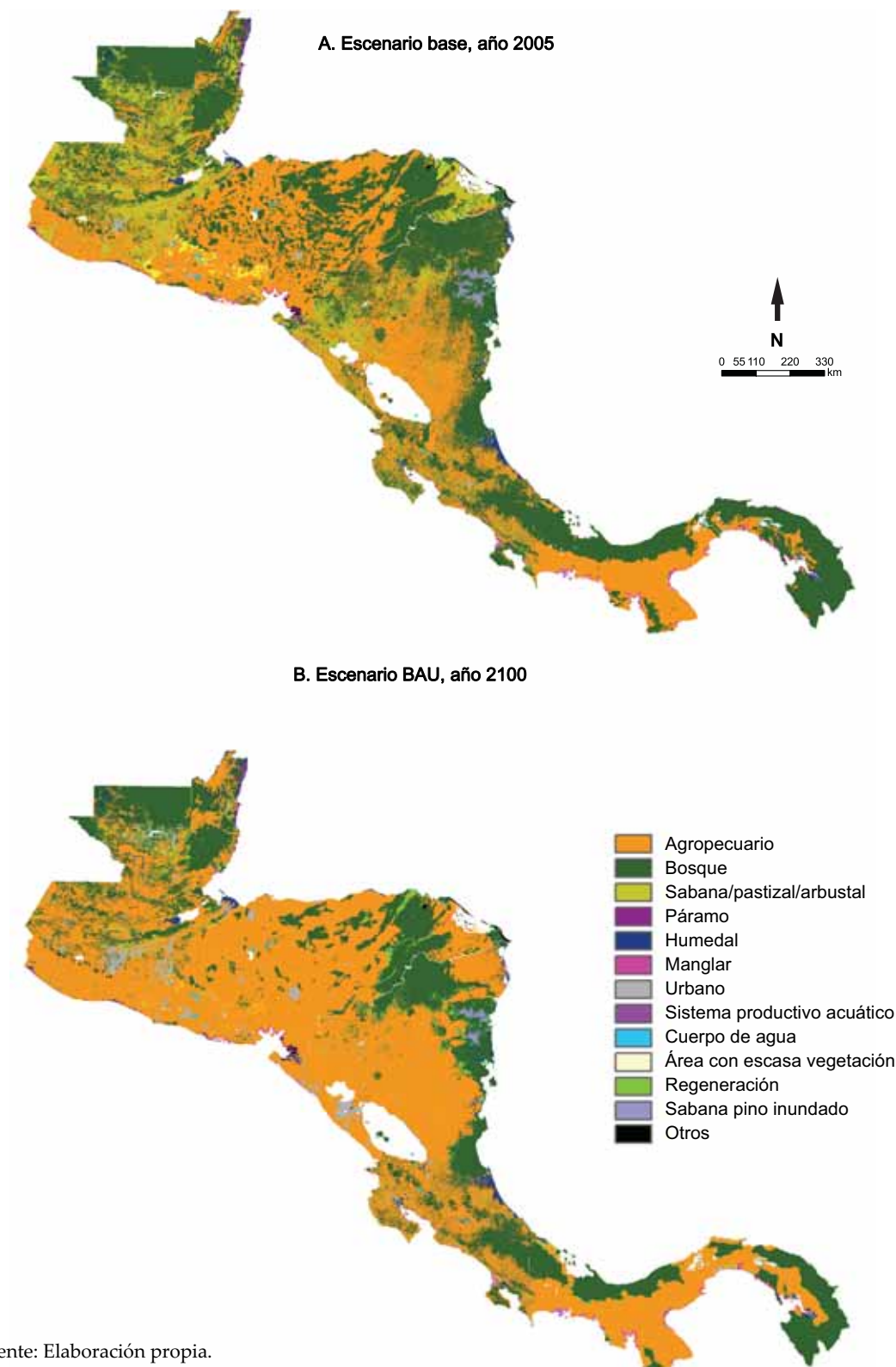
MAPA 3.1 CENTROAMÉRICA: ESCENARIO DE CAMBIO EN USO DE LA TIERRA, 2005 (BASE) Y 2100 (SIN CAMBIO CLIMÁTICO/BAU)
