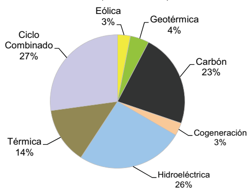
GRÁFICO 8.8 CENTROAMÉRICA: GENERACIÓN DE ENERGÍA ELÉCTRICA, POR TIPO DE TECNOLOGÍA CON ESCENARIO BASE EN 2100 Total = (350.489 GWh)
