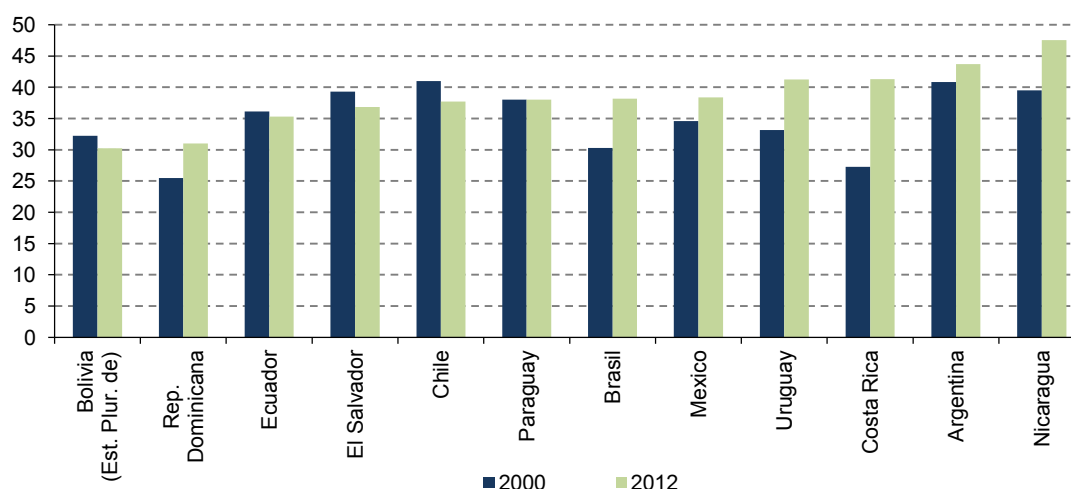
Gráfico 20 Eficiencia de la generación térmica (Porcentajes)
