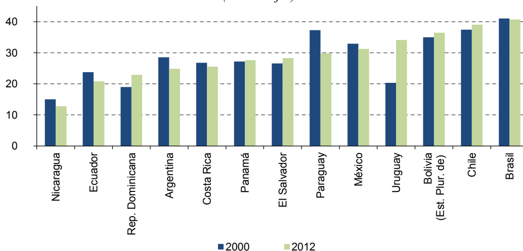
Gráfico 57 Participación de la industria en el consumo final de energía (Porcentajes)
