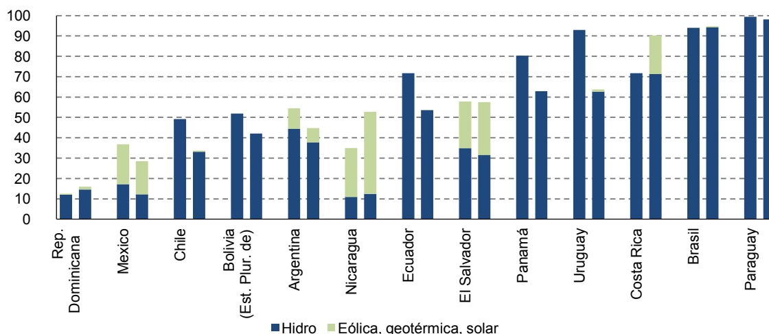
Gráfico 21 Participación de las renovables en la generación eléctrica, 2000-2012 (Porcentajes)
