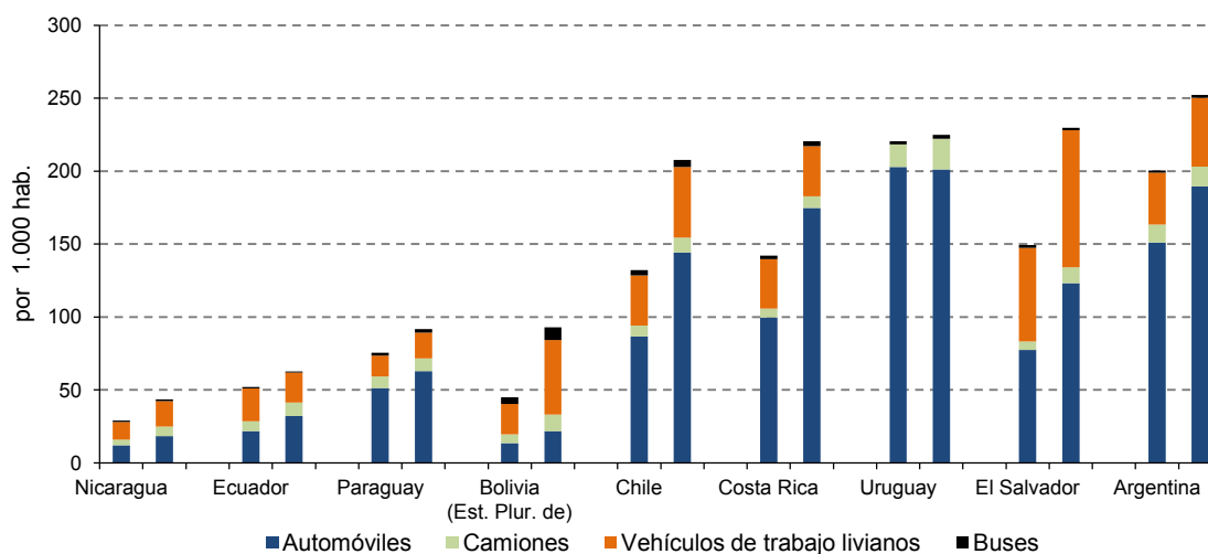
Gráfico 47 Parque vehicular (2000, 2012) (Por 1.000 hab.)
