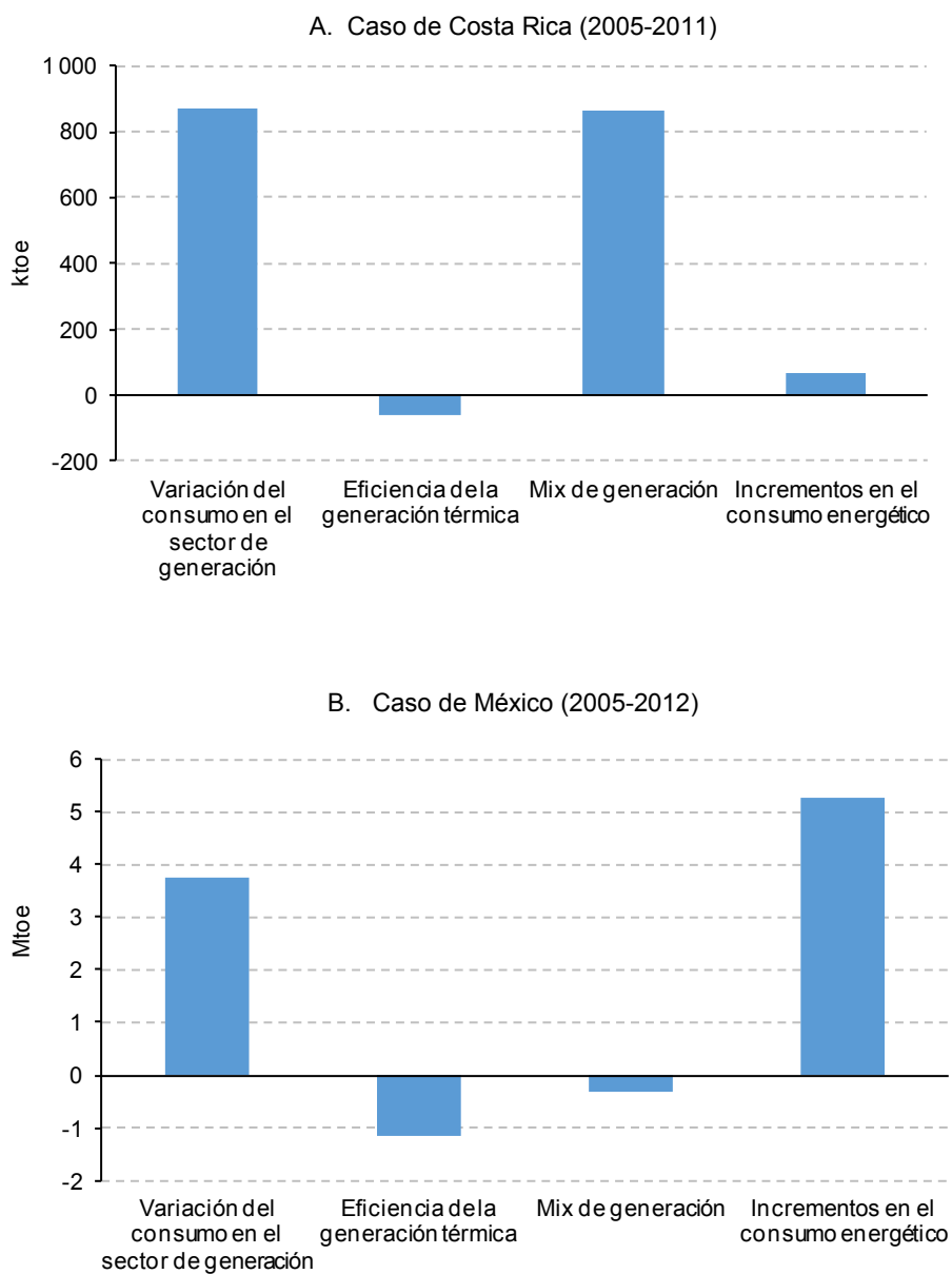
Gráfico 22 Descomposición de la variación en el consumo del sector generación (Ktbe / Mtbe)
