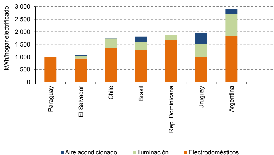
Gráfico 39 Consumo eléctrico específico para electrodomésticos, iluminación y refrigeración a (Kwh)
