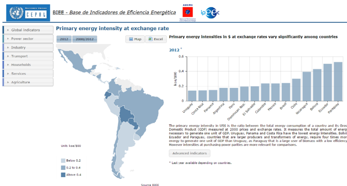
Diagrama 2 BIEE – Base de Indicadores de Eficiencia Energética
