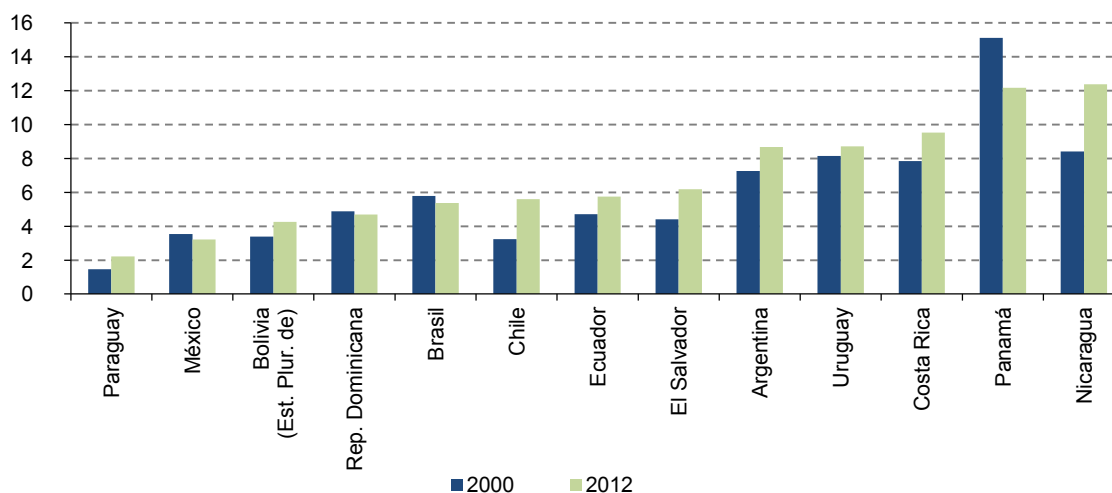
Gráfico 67 Participación del sector servicios en el consumo final de energía
