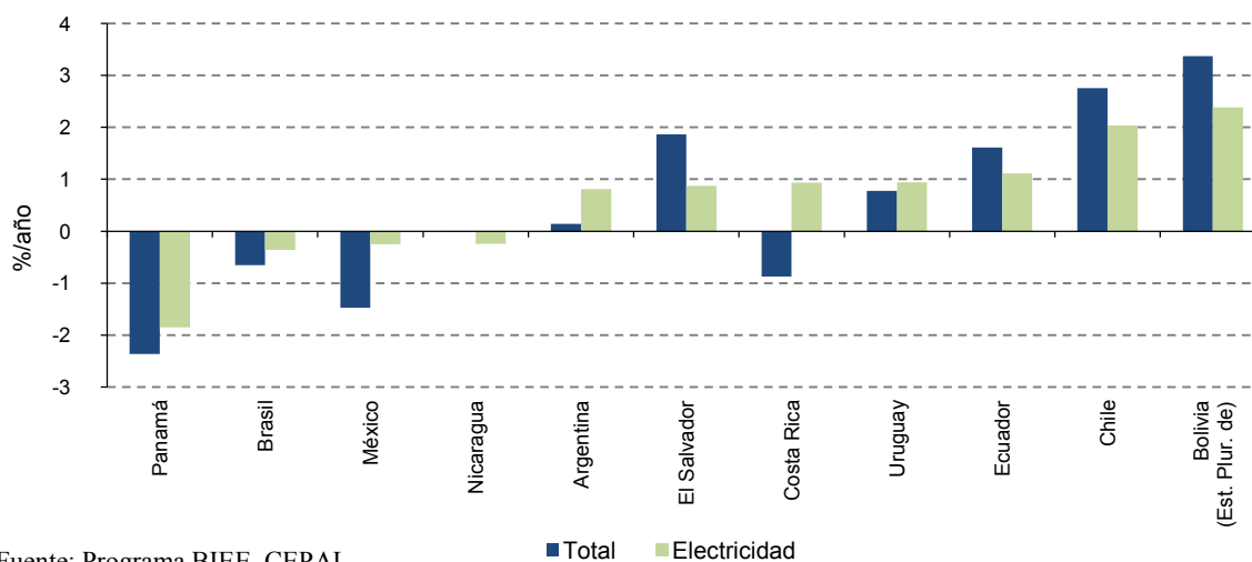
Gráfico 71 Tendencias en la intensidad energética del sector servicios, 2000-2012 (Porcentajes)
