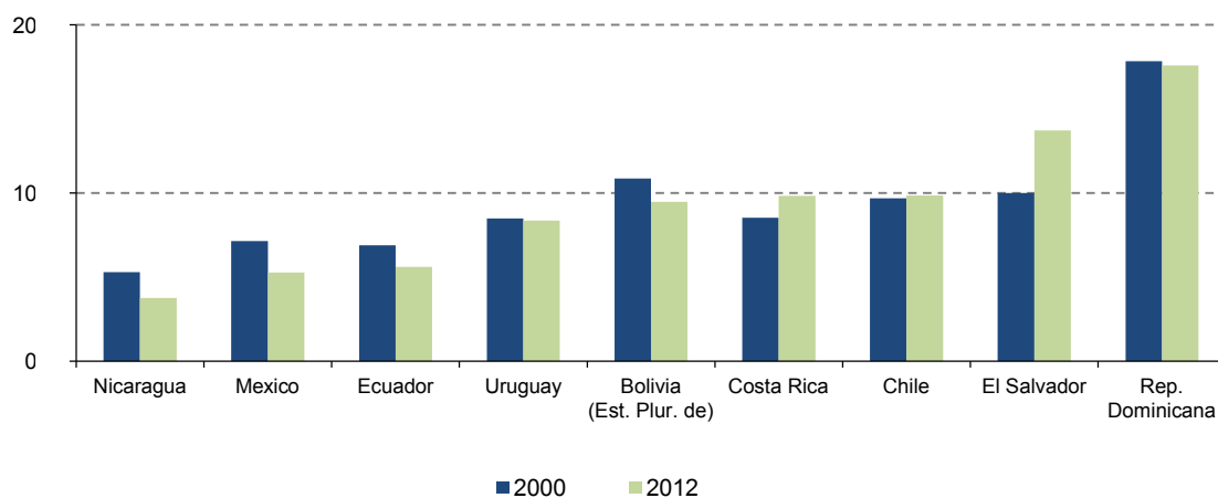
Gráfico 53 Participación del transporte aéreo en el consumo energético del sector transporte (Porcentajes)
