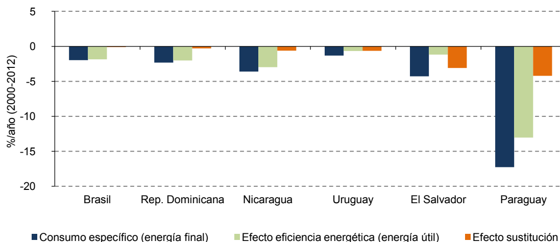
Gráfico 36 Consumo para cocción por vivienda y sustitución (Porcentajes)
