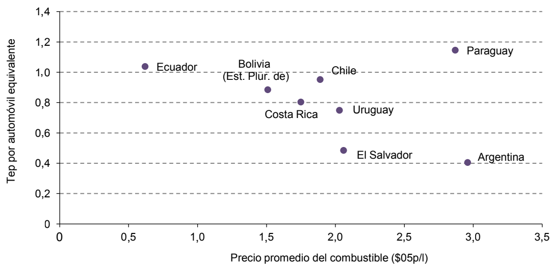
Gráfico 50 Consumo por vehículo equivalente y precios de combustibles vehiculares, 2012
