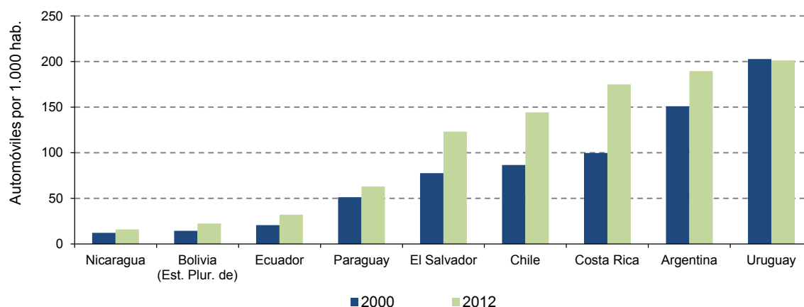
Gráfico 48 Número de automóviles por 1.000 habitantes (Automóviles por 1.000 hab)
