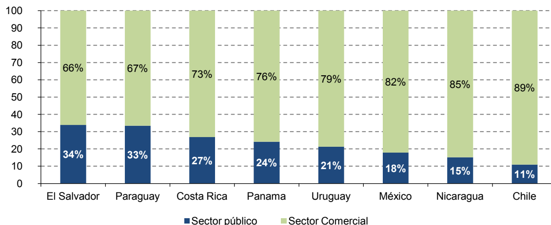
Gráfico 68 Consumo energético de los servicios por rama (Porcentajes)
