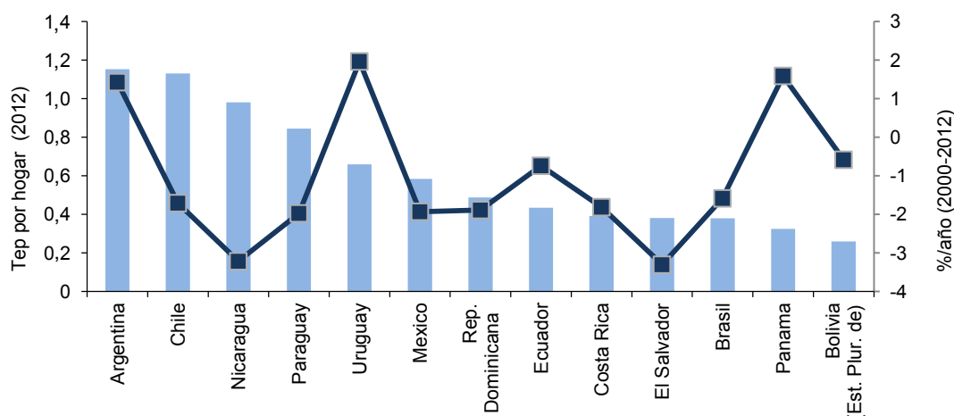
Gráfico 28 Consumo promedio de energía por hogar (Tep/hogar y Porcentajes)
