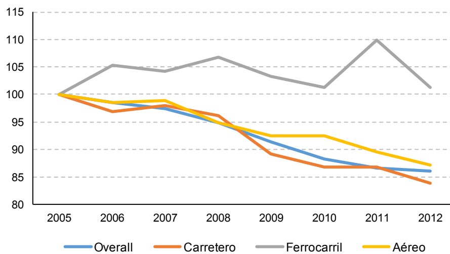
Gráfico 56 Tendencias en la eficiencia energética del transporte en México en base a ODEX
