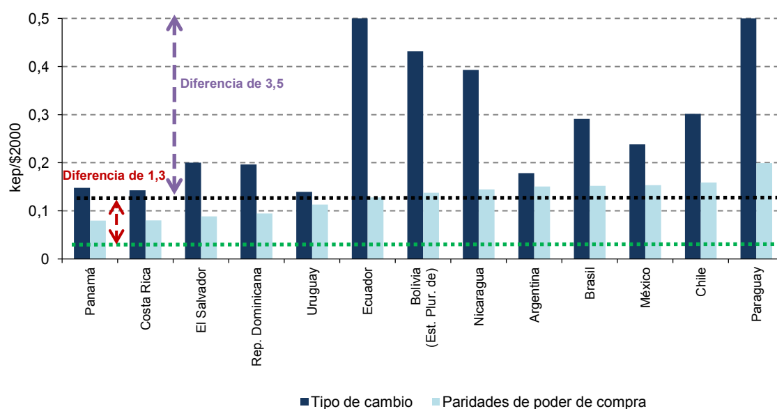
Gráfico 10 Intensidad primaria de energía: tipo de cambio versus paridad de poder de compra, 2012 (Kep/$2000)
