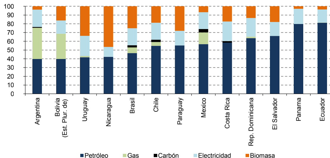
Gráfico 6 Consumo final, desgregado por fuente de energía (2012) (Porcentajes)
