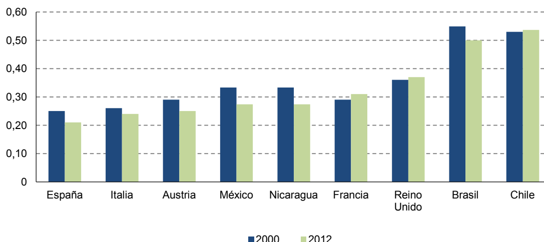
Gráfico 65 Tendencias de consumo específico en la industria del acero, 2000-2012
