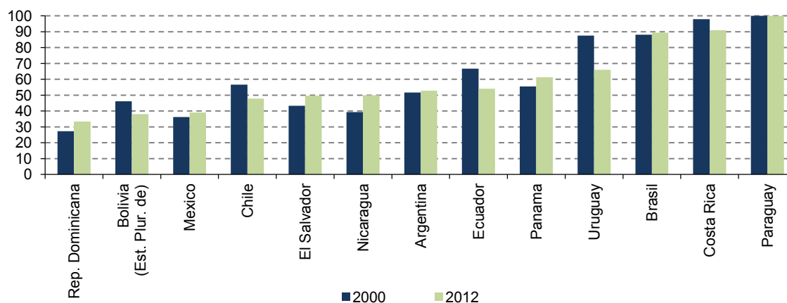
Gráfico 19 Eficiencia en la generación eléctrica (Porcentajes)
