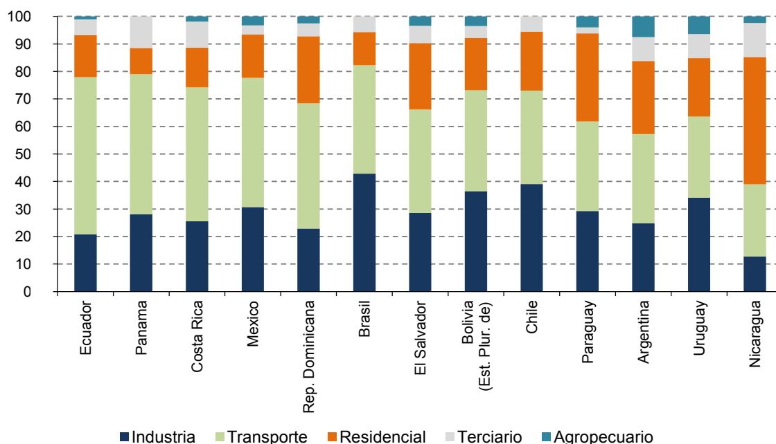
Gráfico 5 Consumo final de energía, desgregado por sector, 2012 a (Porcentajes)
