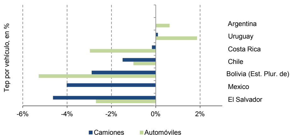
Gráfico 52 Tendencias de consumo para el transporte carretero por tipo de vehículo 2000 y 2012 (Porcentajes)
