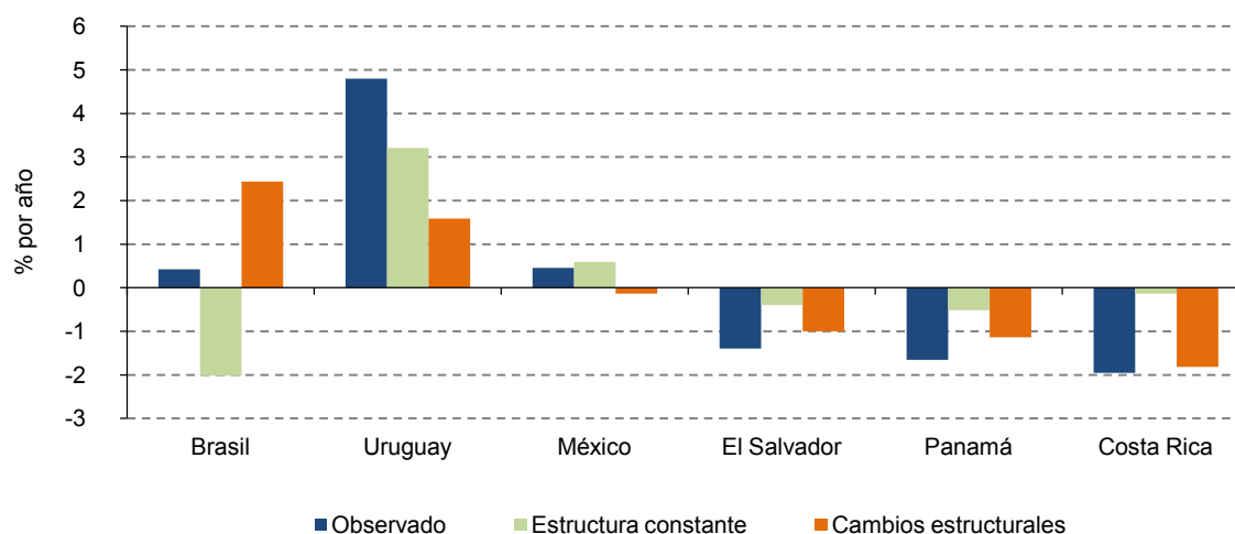
Gráfico 63 Efecto estructural en las industrias manufactureras, 2000-2012 (Porcentajes)
