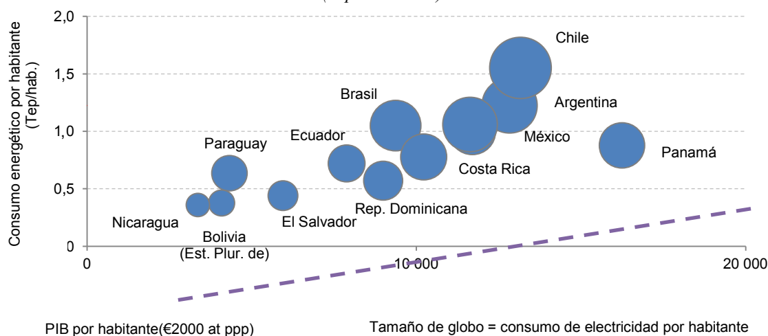
Gráfico 9 Consumo final de energía y PIB per cápita (2012) (Tep/habitantes)
