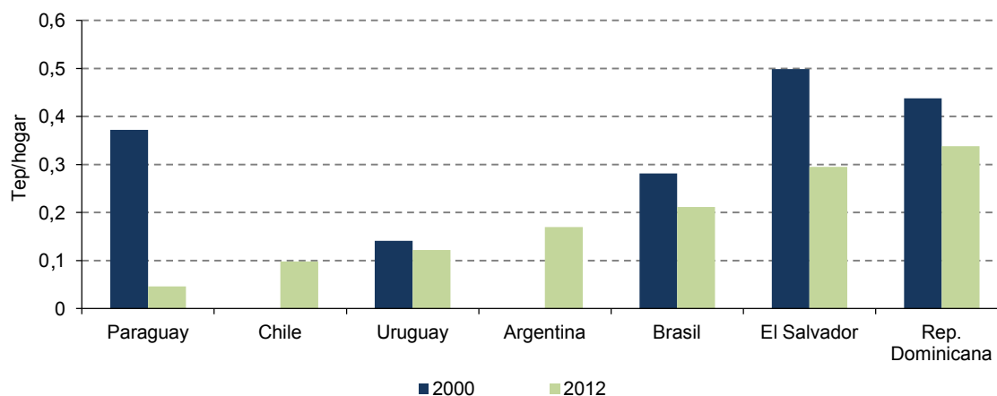
Gráfico 35 Consumo unitario en cocción por hogar (Tep/hogar)
