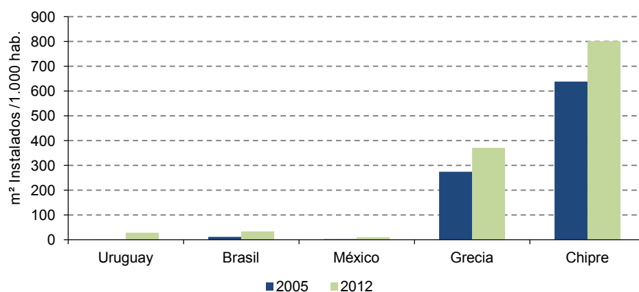
Gráfico 38 Tasa de equipamiento de los hogares con calentadores de agua solares: comparación con países de la UE (Mts 2 )
