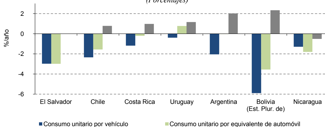
Gráfico 49 Tendencias en el consumo del transporte carretero, 2000-2012 (Porcentajes)
