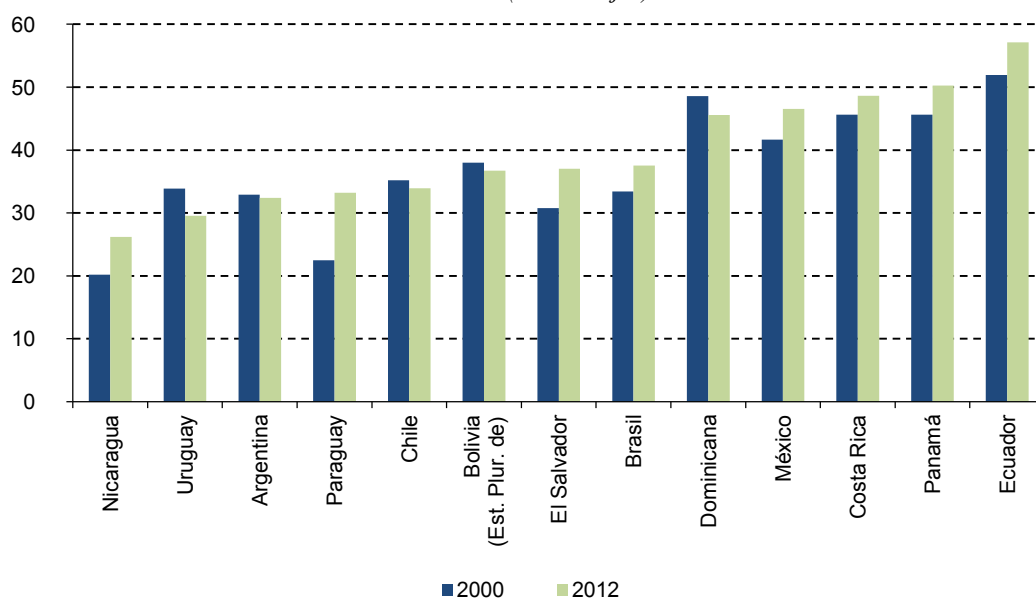
Gráfico 44 Participación del sector transporte en el consumo final de energía (Porcentajes)
