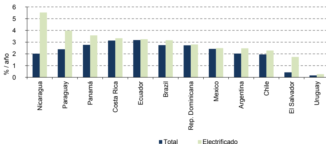
Gráfico 26 Tendencias en el número de hogares: total y electrificado, 2000-2012 (Porcentajes)
