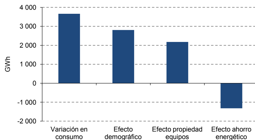
Gráfico 42 Fuerzas que impulsan la variación en el consumo de los refrigeradores en Brasil, 2005-2012 a (Gwh)
