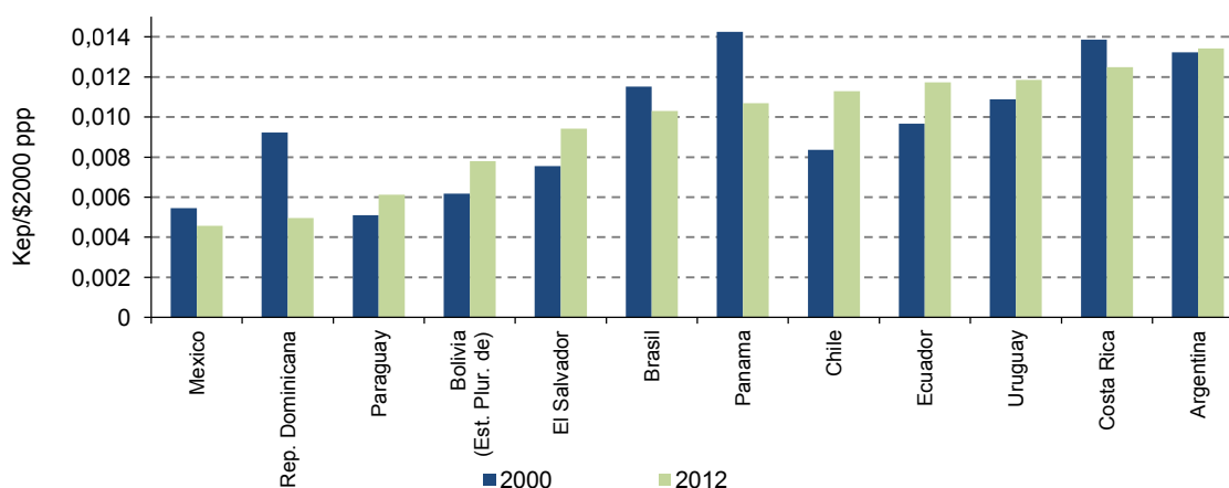
Gráfico 70 Intensidad energética del sector servicios
