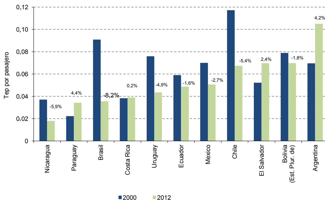
Gráfico 54 Consumo unitario del transporte aéreo por pasajero a (Tep/pasajero y Porcentajes)
