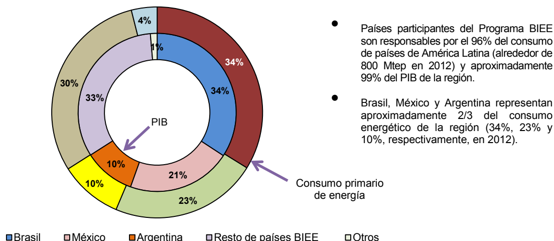
Gráfico 1 Consumo primario de energía y PIB en América Latina, 2012 (Porcentajes)
