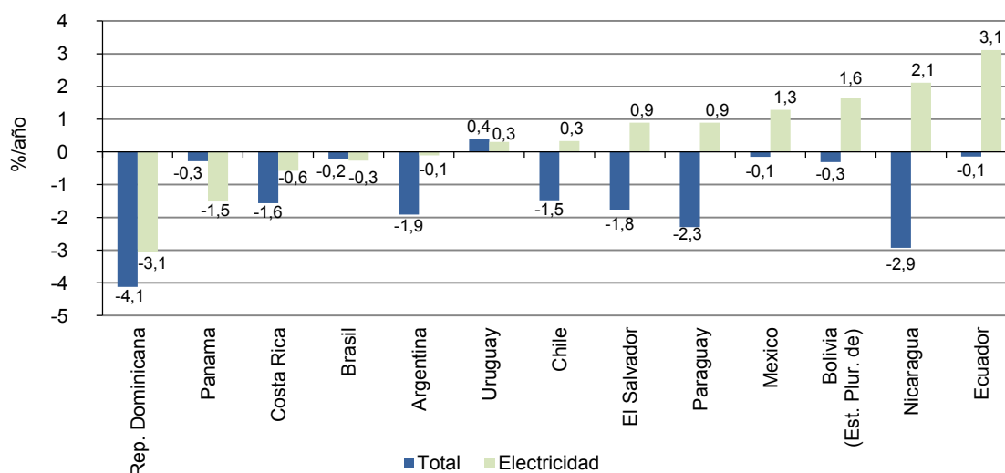
Gráfico 14 Tendencias de intensidad energética final: total y electricidad, 2000-2012 (Porcentajes)
