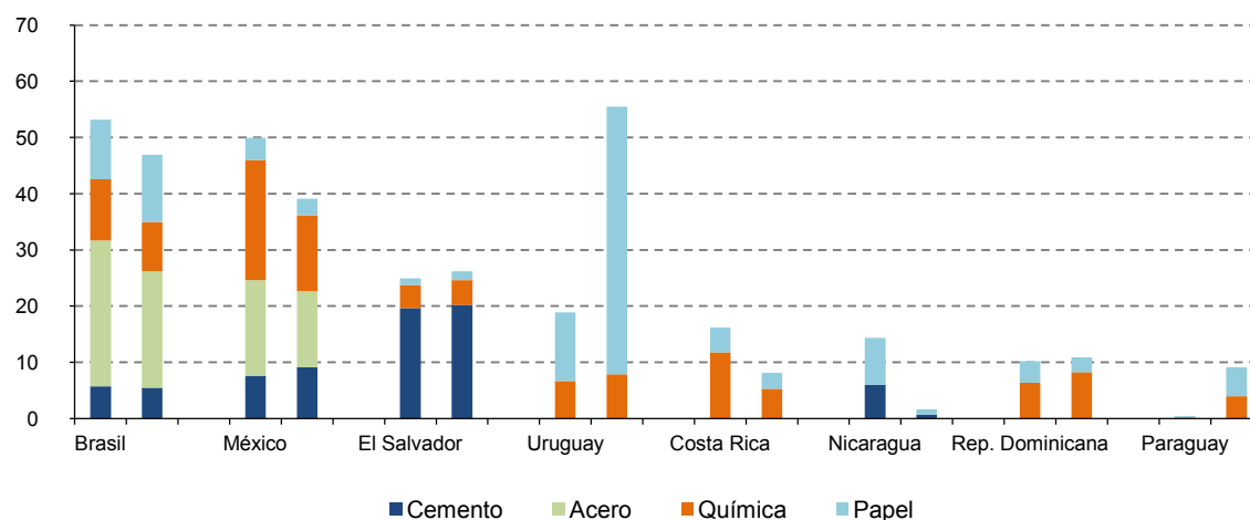
Gráfico 60 Ramas de actividad industrial con alta intensidad energética, 2000-2012 (Porcentajes)
