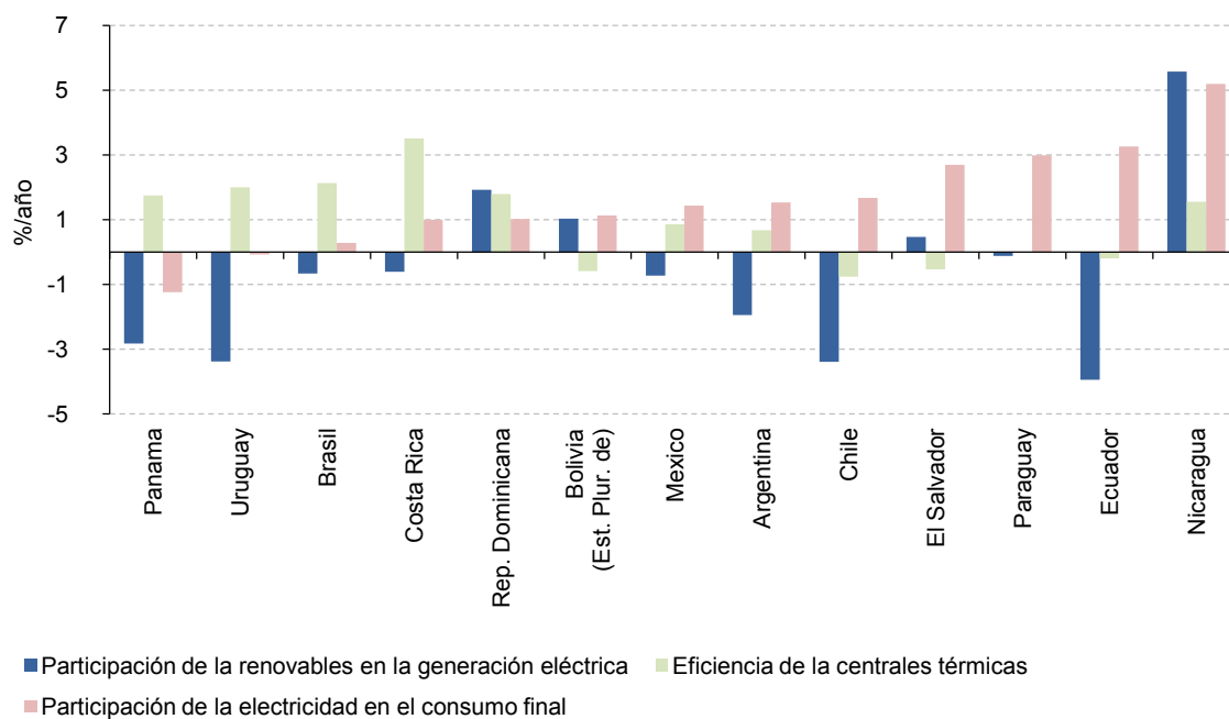
Gráfico 13 Participación de las energías renovables en la generación eléctrica, eficiencia de energía térmica y la penetración eléctrica (Porcentajes)
