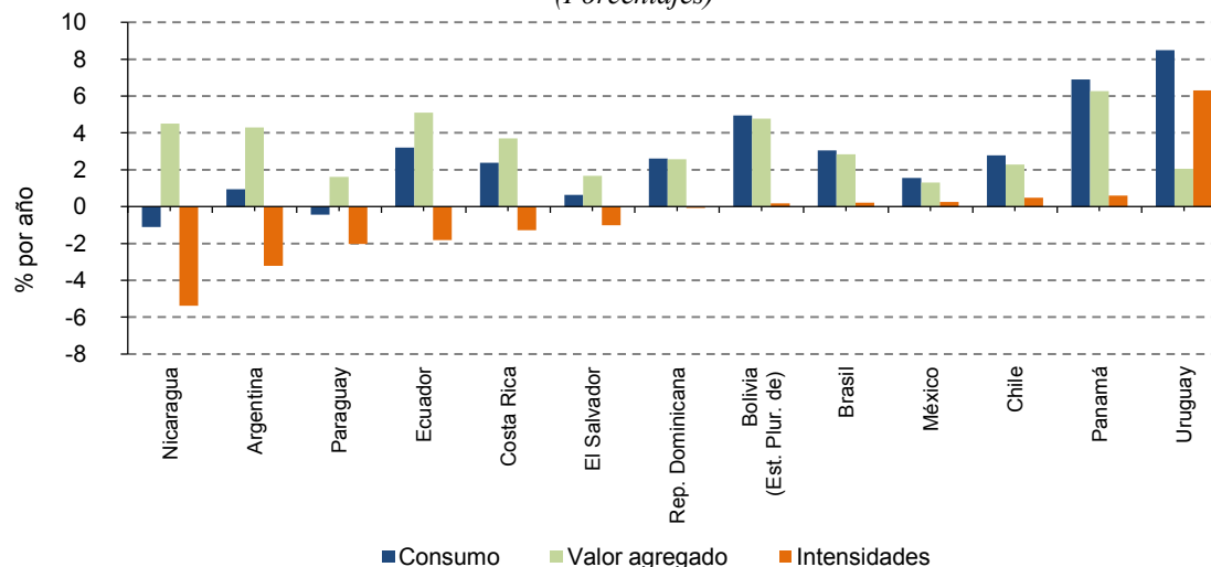
Gráfico 59 Tendencias de intensidad energética en el sector industrial, 2000-2012 (Porcentajes)
