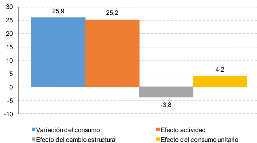
Gráfico 66 Descomposición de la variación en el consumo industrial de energía en Brasil, 2000-2011
