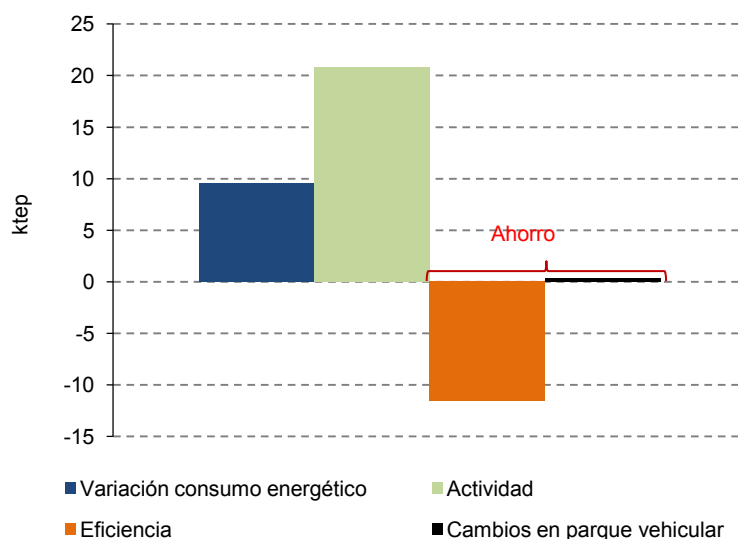
Gráfico 55 Descomposición del consumo del sector transporte: caso de México, 2005-2012 (Ktep)
