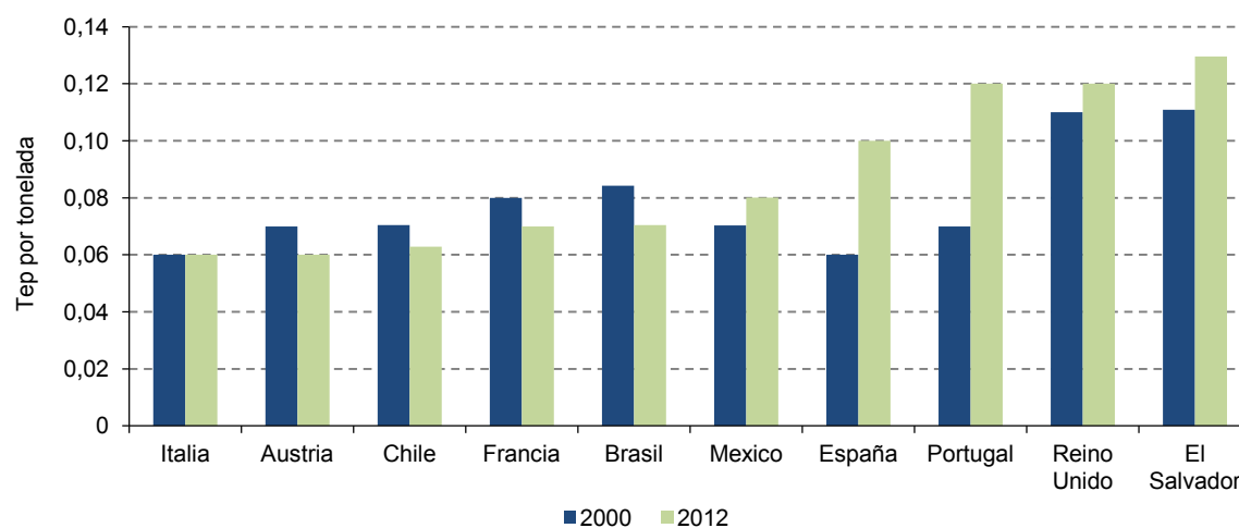
Gráfico 64 Tendencias de consumo específico en la industria del cemento, 2000-2012
