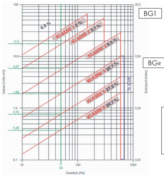
Figura 8.10. Resultados de bandas pre-comprimidas según EN 12207.
