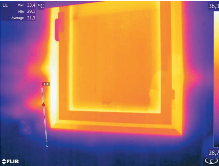
Foto 11.24. Entradas de aire caliente exterior. En verano las entradas de aire en la vivienda se ven con un patrón térmico diferente al de invierno, sobre todo si la fachada está soleada en ese momento.
