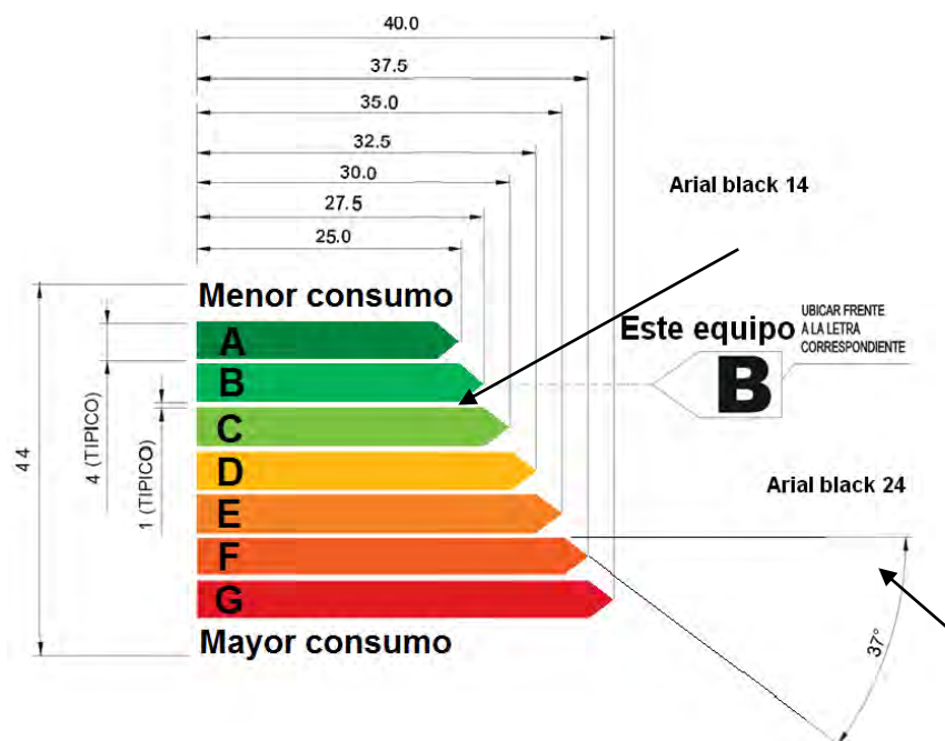
Figura 6.3.3.1. Especificaciones para la ilustración de rangos de eficiencia con barras de colores en tamaño de etiqueta A6 (Dimensiones en milímetros).
